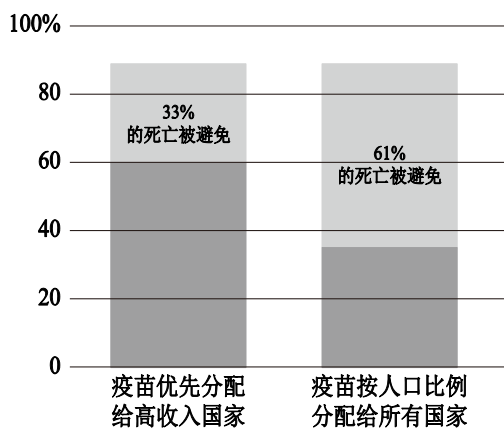
图 5 模型推演的新冠肺炎疫情死亡人数占比（与没有疫苗状态相比）
